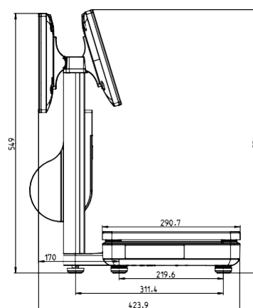
Zboku (11,6-palcový displej zákazníka)
