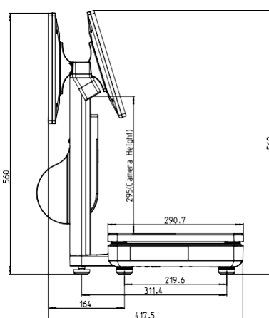
Zboku (15,6-palcový displej zákazníka)
