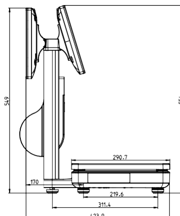
Zijkant (11,6-inch klantendisplay)
