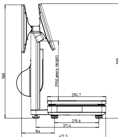
Zijkant (15,6-inch klantendisplay)
