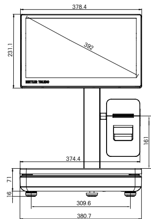
正视图
