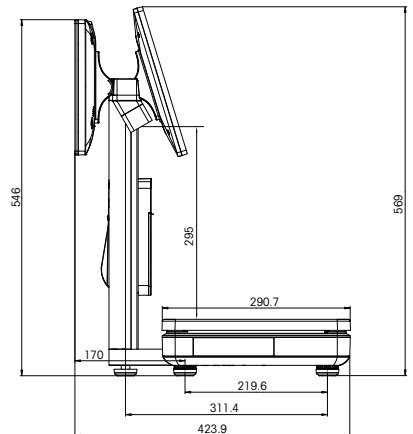
侧视图(11.6英寸客显版本)
