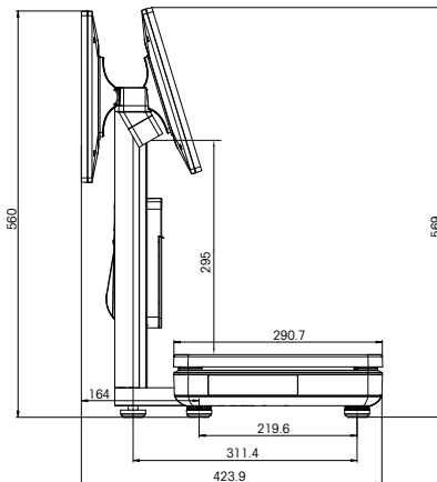
侧视图(15.6英寸客显版本)
